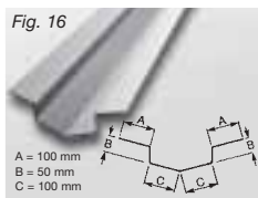
Fig. 16 A = 100 mm B = 50 mm C = 100 mm Försänkt rännal
