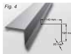
Fig. 4 Gavelbeslag 1
