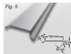
Fig. 5 Vindskivebeslag
