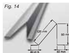
Fig. 14 Snörasskydd
