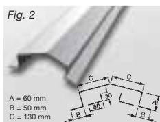
Fig. 2 A = 60 mm B = 50 mm C = 130 mm Ventilerad nock
