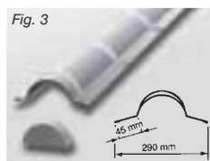
Fig. 3 Nockpanna - Ändstycke
