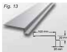
Fig. 13 Foderbeslag
