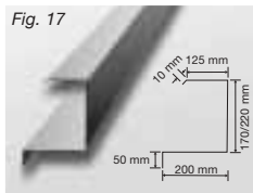
Fig. 17 Gavelbeslag 2
