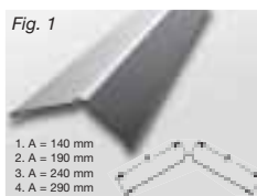
Fig. 1 1. A = 140 mm 2. A = 190 mm 3. A = 240 mm 4. A = 290 mm Nockplåt
