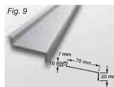
Fig. 9 Fönsterbleck
