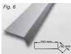
Fig. 6 Fotplåt
