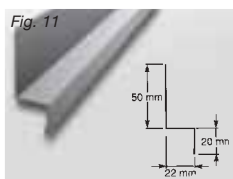
Fig. 11 Sockelbeslag
